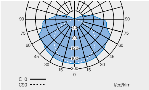
Polar curve nLLK 09036 / nLLK 09058
